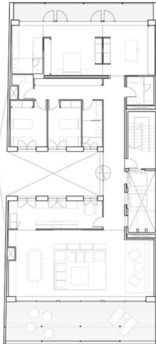
PLANTA 8 (Ático)
